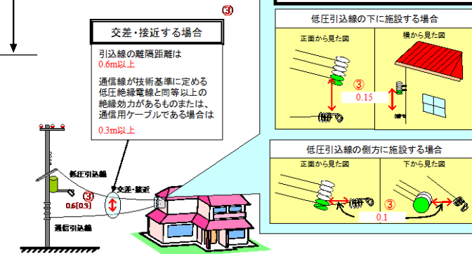
交差・接近する場合の弊社低圧引込線と事業者様通信線との離隔距離
