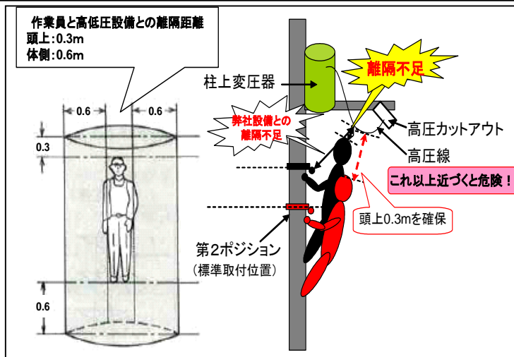
作業員と弊社設備との離隔距離
